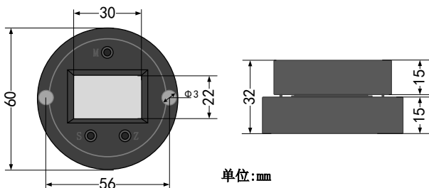
图 2 MS0110 尺寸
