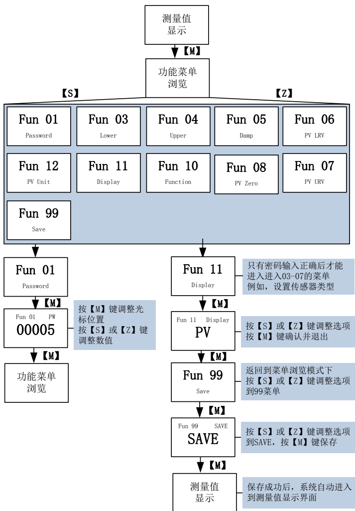
图 14 功能切换图
