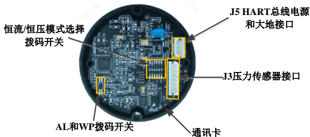
图 3 硬件接口说明
