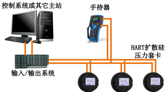
图 8 HART 组网模式
