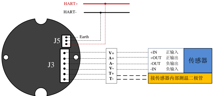
图 4 MS0110 接线示意图
