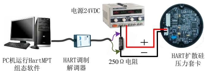
图6 系统连接示意图
