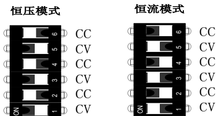
图5 传感器供电模式选择拨码开关
