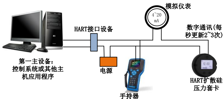
图 7 (4~20)mA 兼容模式
