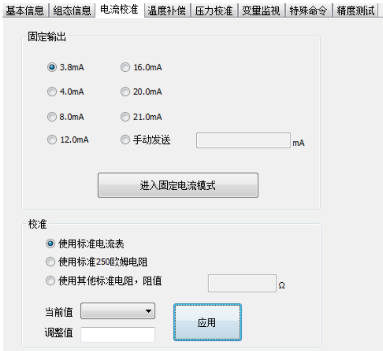
图 11 电流校准
