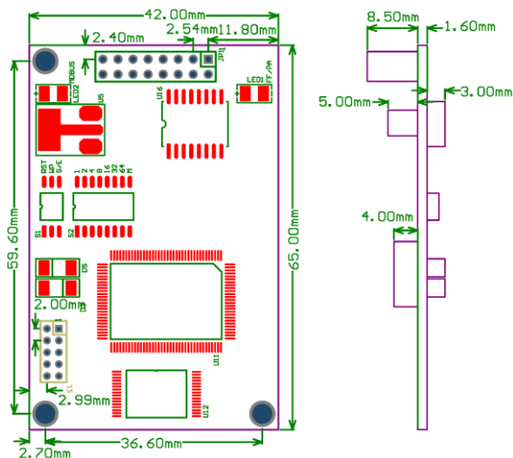
图 1.2 嵌入式模块设备外型尺寸（单位：mm）
