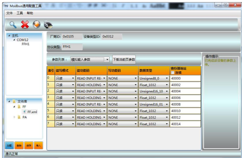
图 4.5 参数配置
