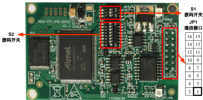
图 2.1 M0313 Modbus 转 FF 嵌入式模块通信接口定义 JP1 通信接口的具体含义如下：
