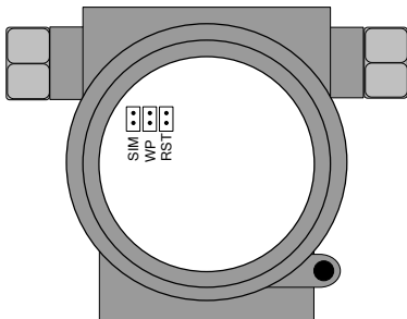
图 7.12 PA 型智能变送器硬件跳线
