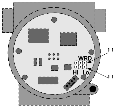
图 5.8 HART 型智能压力变送器硬件跳线
