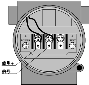
图 2.3 FF、PA 型智能变送器接线图
