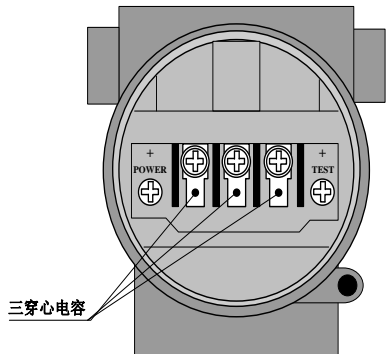
图 3.4 穿心电容的位置
