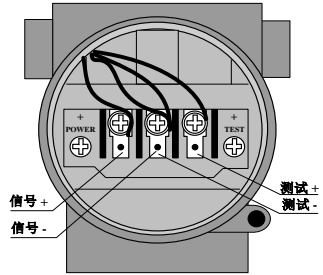
图 2.4 HART 型智能变送器接线图
