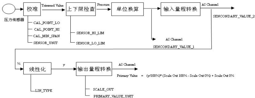
图 7.3 变换块结构
