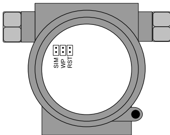
图 6.7 FF 智能压力变送器硬件跳线
