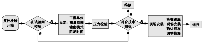
图 2.5 智能变送器复校检验流程
