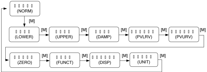
图4.2 调整功能切换图
