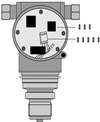
图 3.5 仪表卡与通讯卡连接
