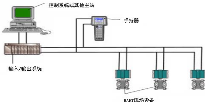
图 5.2 HART 多点接线方式
