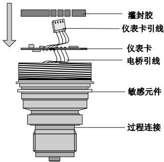
图 3.3 传感器与仪表卡
