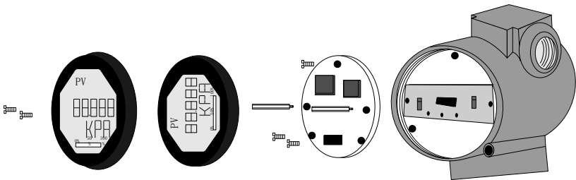
图 3.7 表头安装结构图
