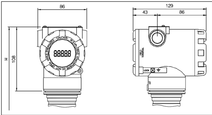
图 1.1 智能变送器外型尺寸（单位：mm）
