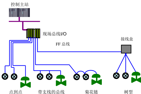
图 6.1 FF 网络拓扑
