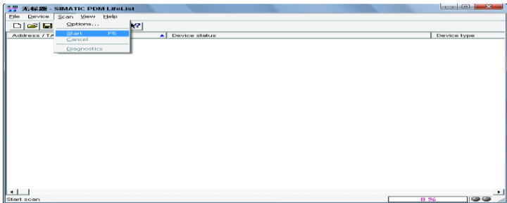
图 7.8 启动 LifeList
